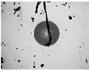
Dirty End Face
